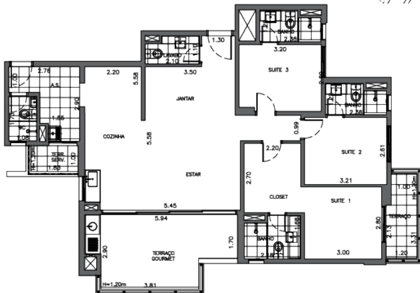
PLANTA 1º AO 20º ANDAR TIPO - FINAL 04 3/ESCALA
