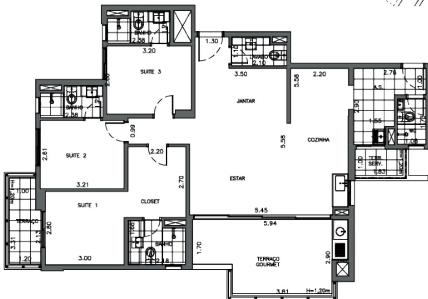
PLANTA 1º AO 20º ANDAR TIPO - FINAL 02 S/ESCALA
